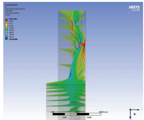
Rys. 10. Model osiowosymetryczny: przypadek obciążenia 2 – naprężenia promieniowe [opracowanie własne]
